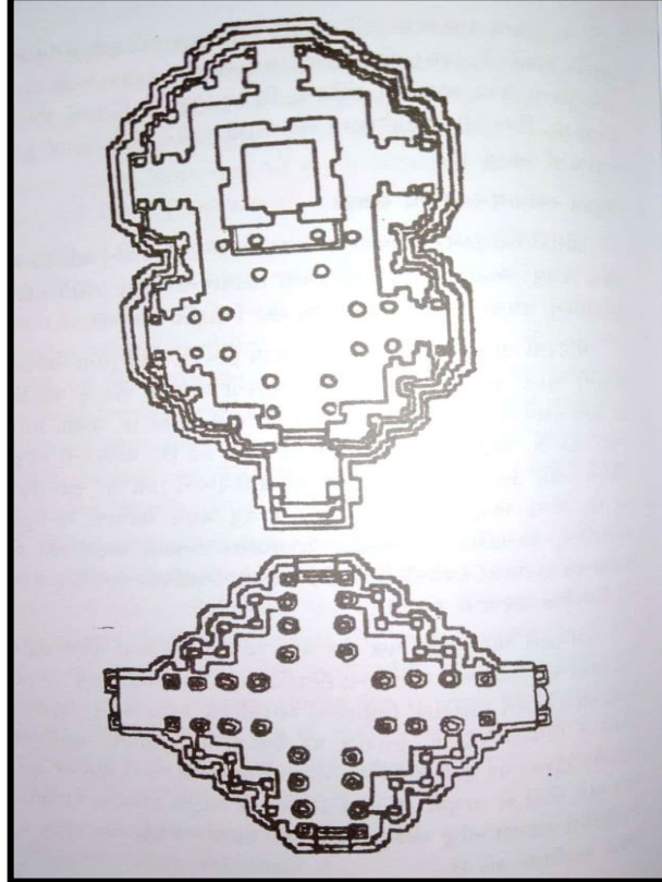
મોઢેરાના મંદિરનું તલમાન
